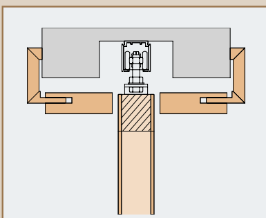
Konstruktionszeichnung Schiebetür in der Wand laufend
