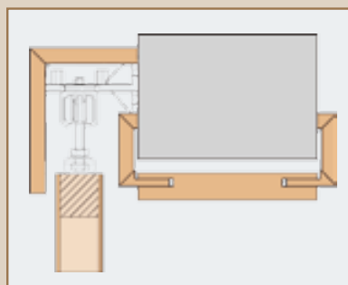
Konstruktionszeichnung Schiebetür vor der Wand laufend
